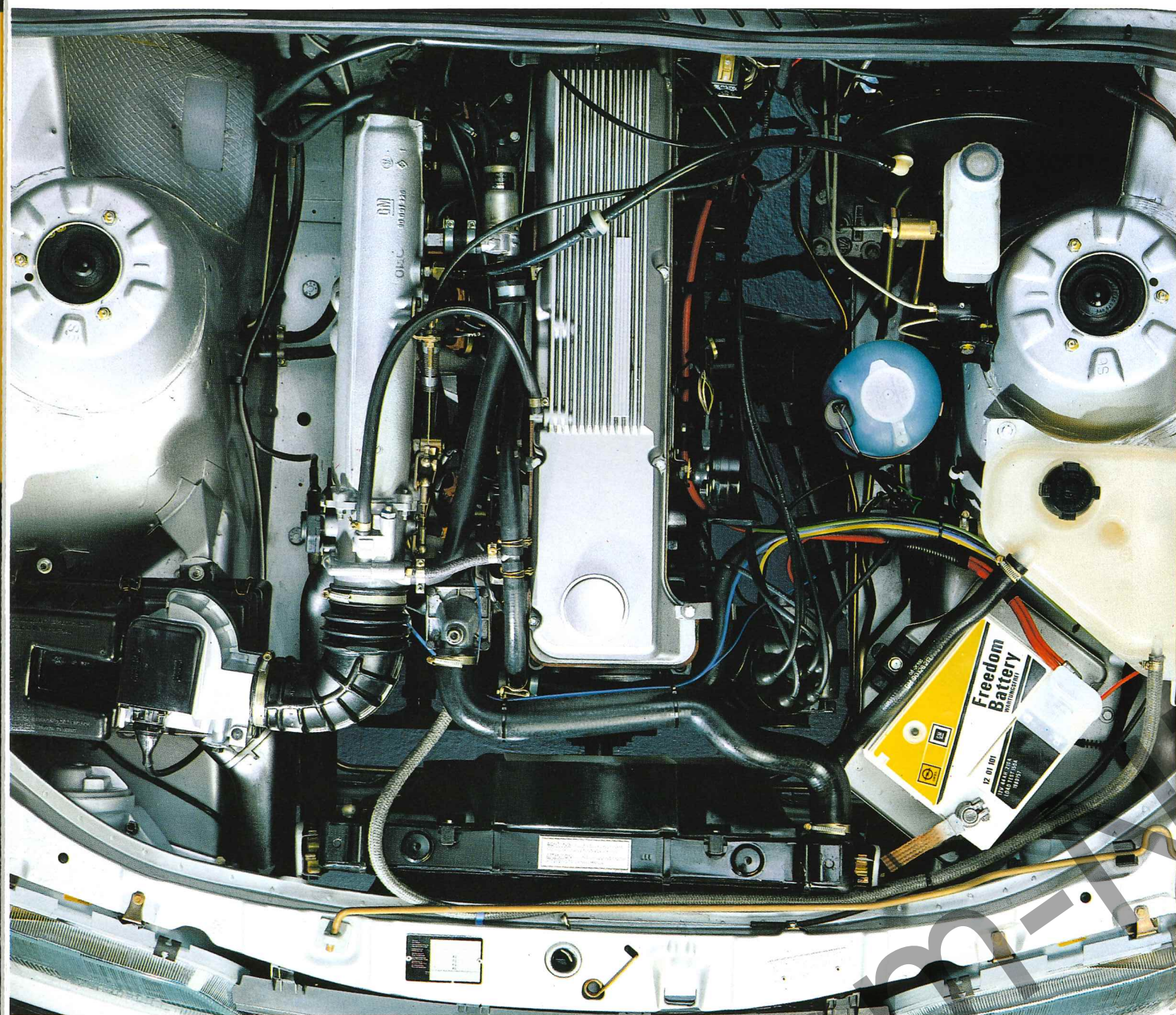
3.0 E-Motor.
